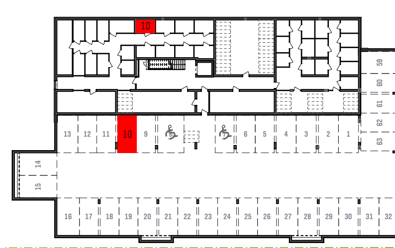
KELLERGESCHOSS | M 1:500
