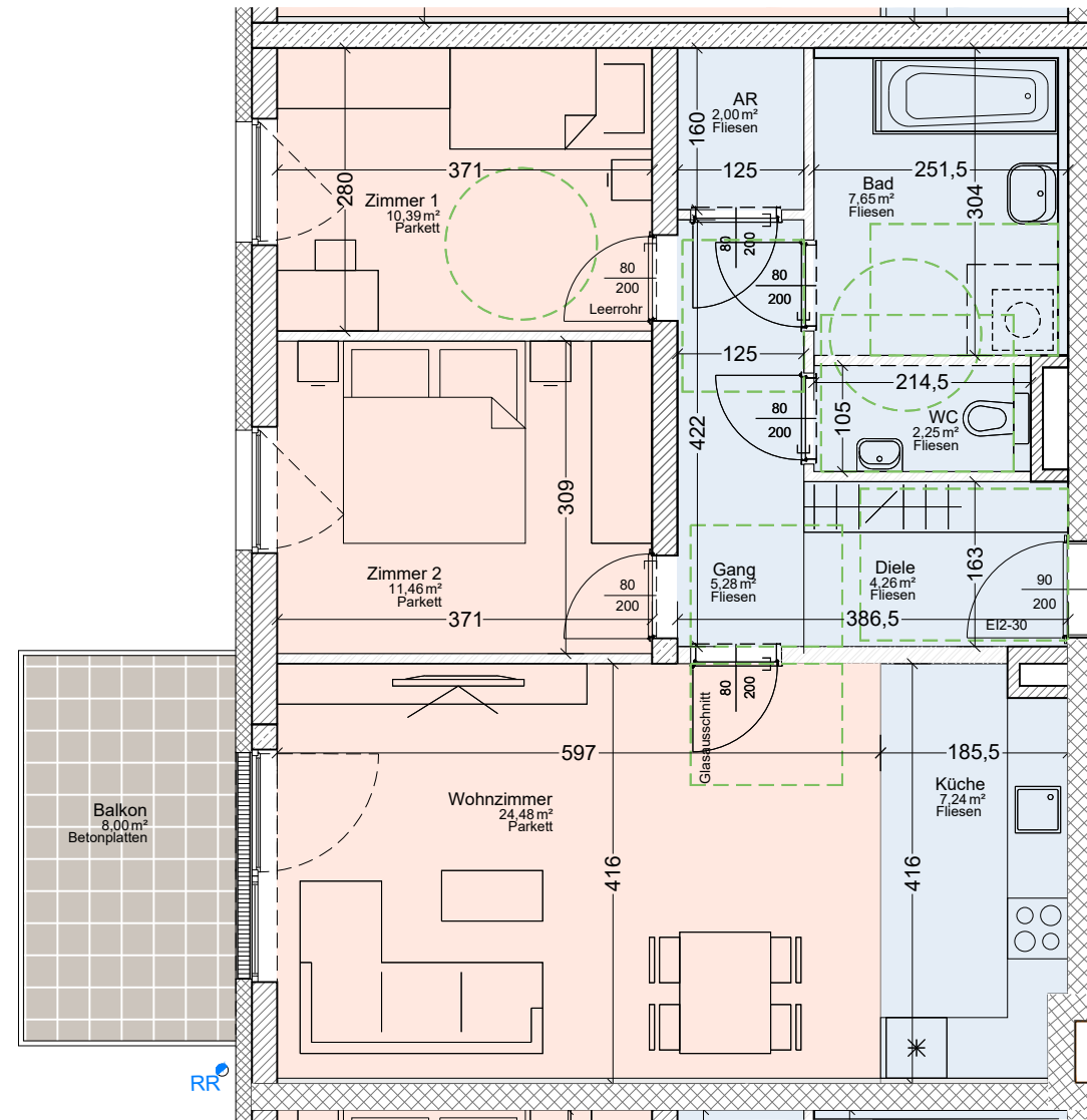
1. OBERGESCHOSS TOP 14 - Tür C11
